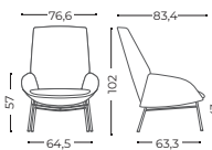
4 Metal legs chair 4 Patas metálicas
