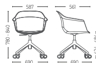
Hollow silent castors Ruedas silenciosas huecas
