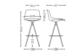
4 Metal legs stool Taburete 4 patas de metal
