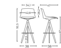
4 Wood legs stool Taburete 4 patas de madera
